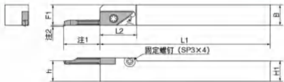
图 1 (SVN-N 型)
