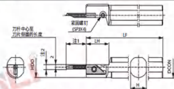
Fig. 2 (S-SVN-SXN)
