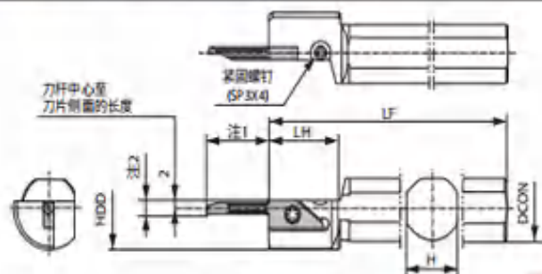
Fig. 1 (S-SVN-XN)
